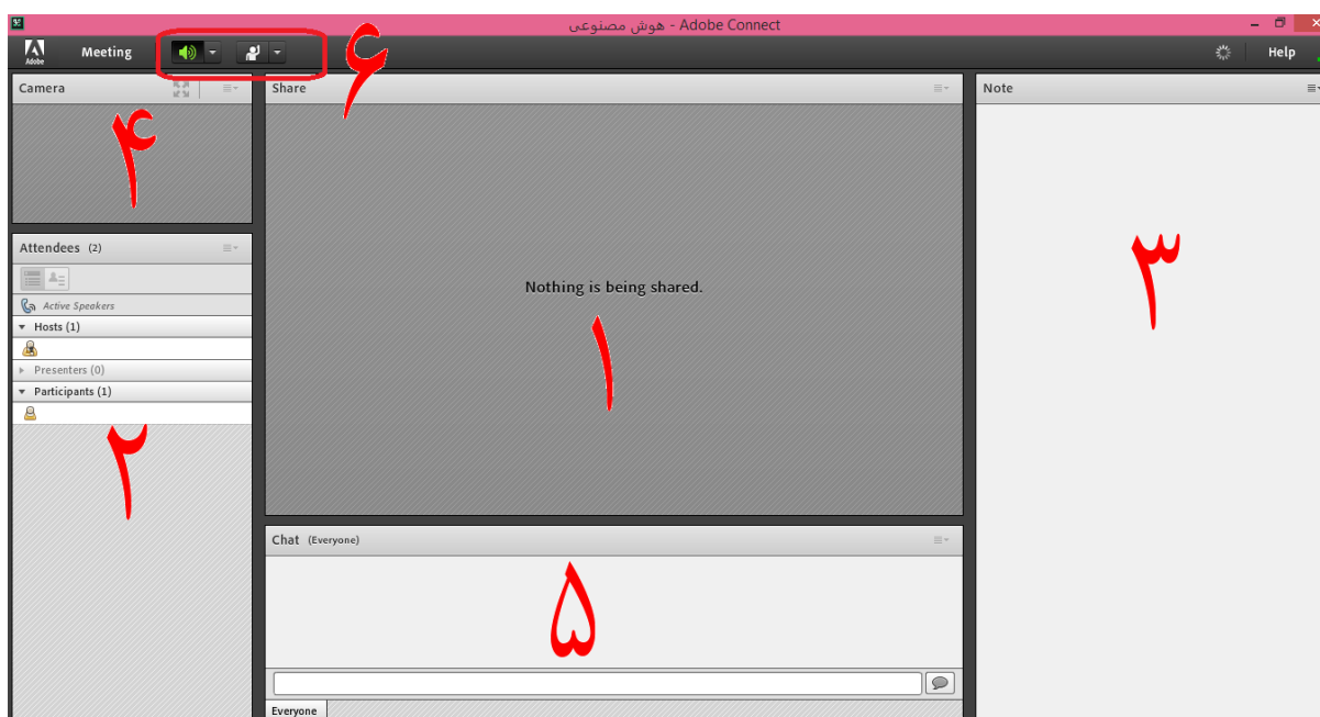
شکل ۲. ساختار کلاس
